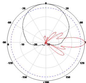
1850~1990MHz: ±45° Pol.
