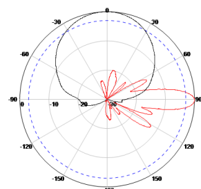
1920~2170MHz: ±45° Pol.
