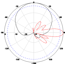
1710~1880MHz: ±45° Pol.
