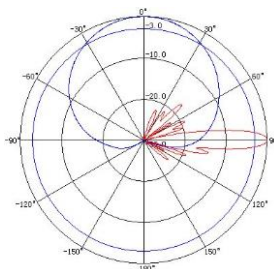
1850~1990MHz: ±45° Pol.
