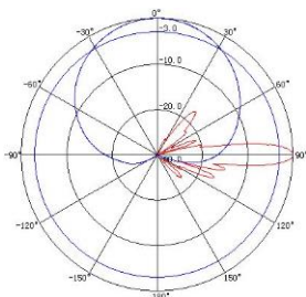
1710~1880MHz: ±45° Pol.
